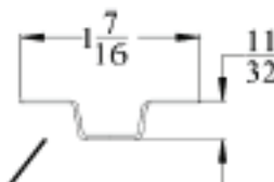
S-2003 22 ga. HDG
